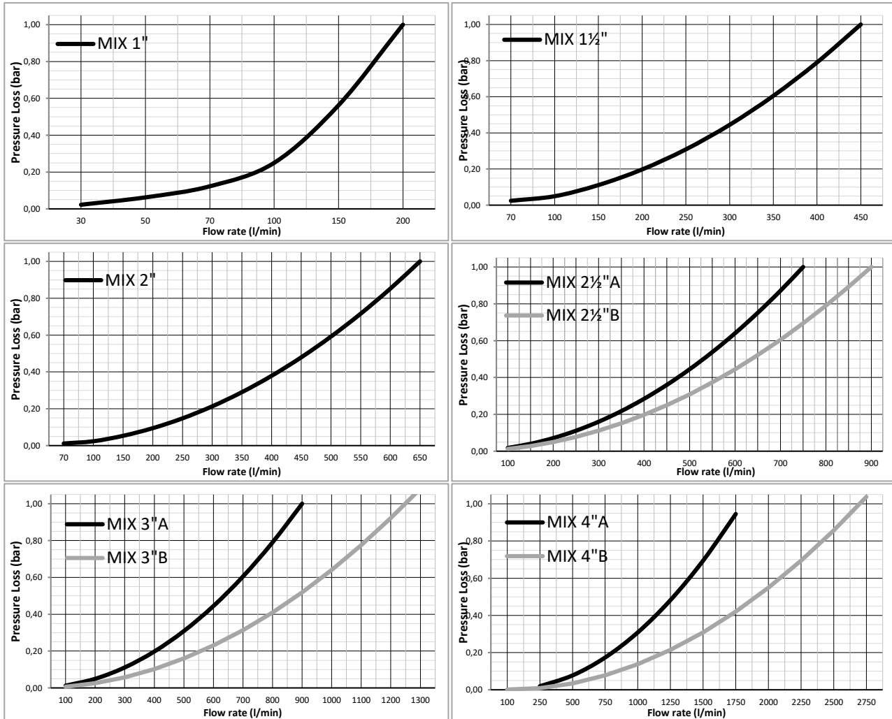
Diagramma perdita di carico – Pressure loss diagram
